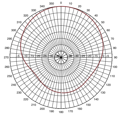
800 MHz H-Plane Pattern
