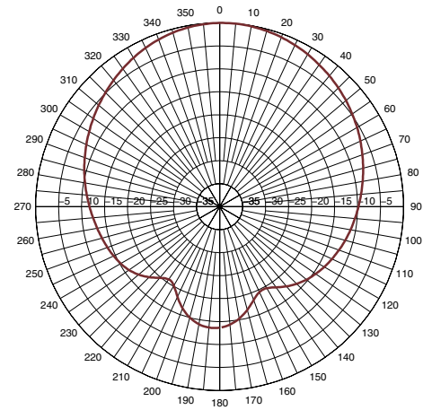
1850 MHz H-Plane Pattern
