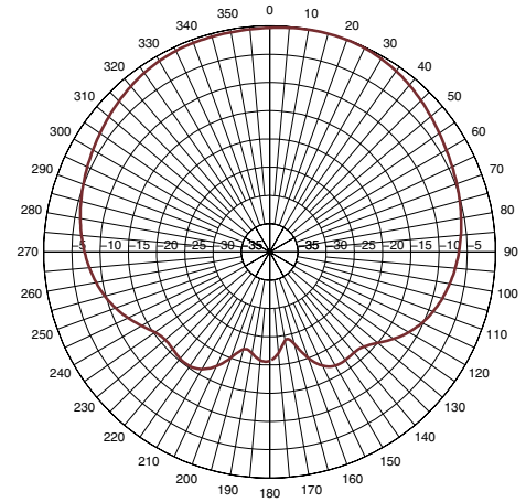
2600 MHz H-Plane Pattern
