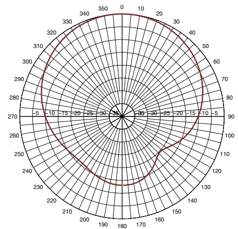
900 MHz H-Plane Pattern
