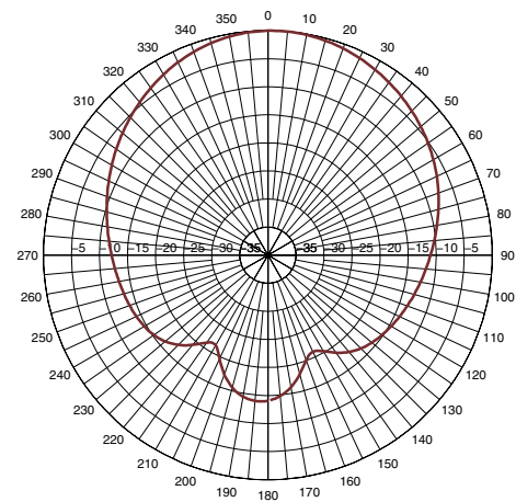
2300 MHz H-Plane Pattern
