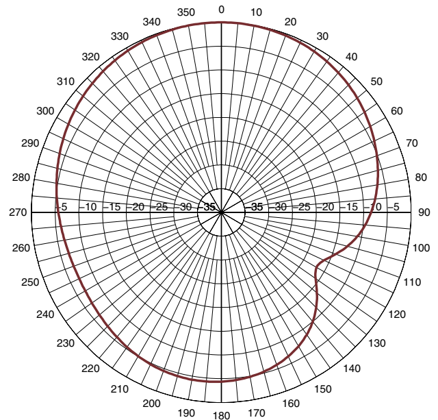
698MHZ_EL
