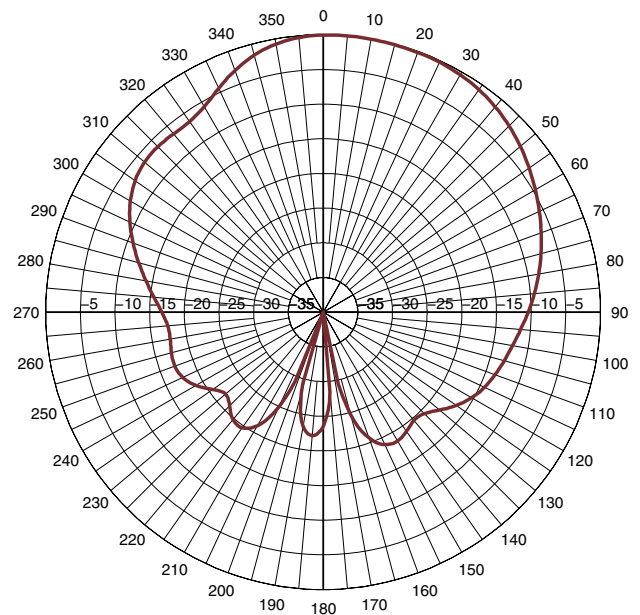
V-PLANE_1710MHZ
