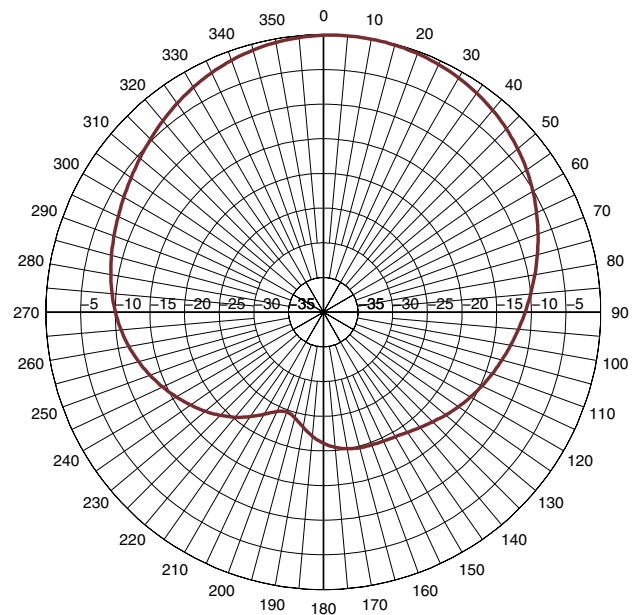
V-PLANE_850MHZ
