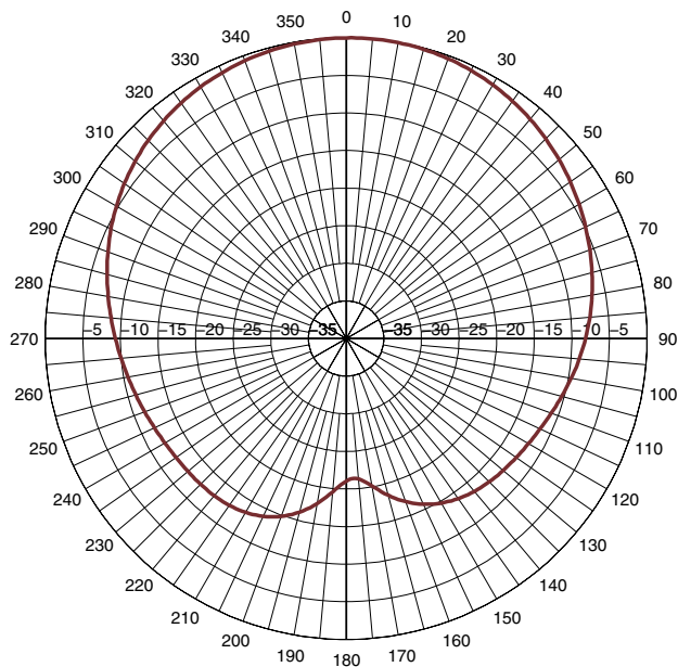
H-PLANE_850MHZ
