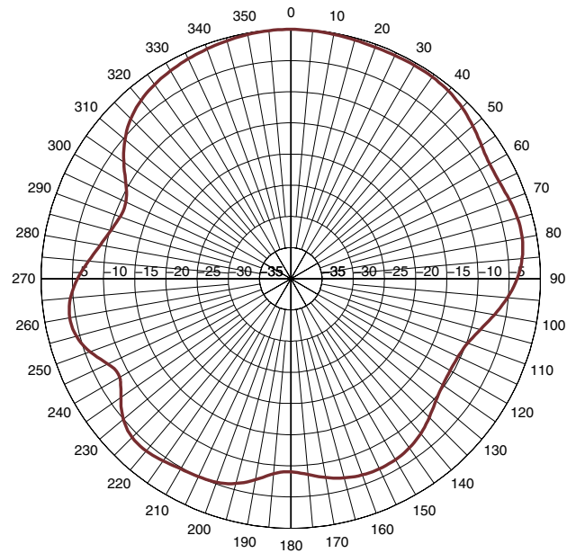
V-PLANE_960MHZ
