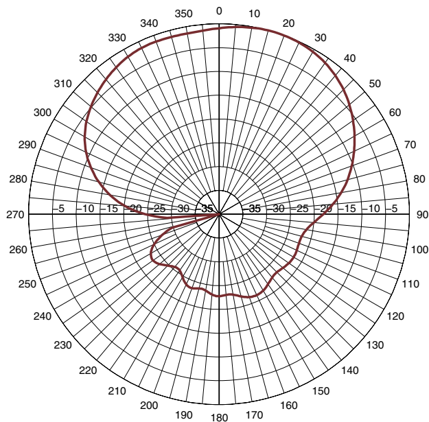
H-PLANE_2700MHZ
