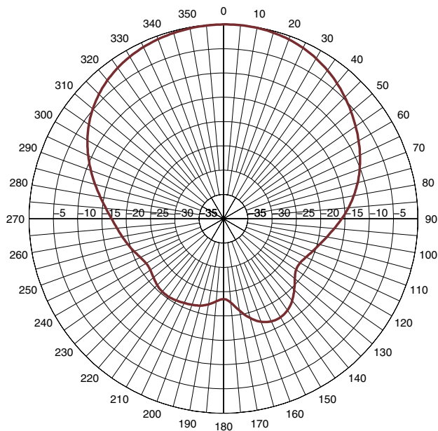
H-PLANE_1710MHZ
