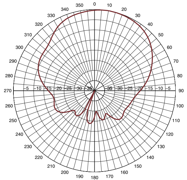
V-PLANE_2100MHZ
