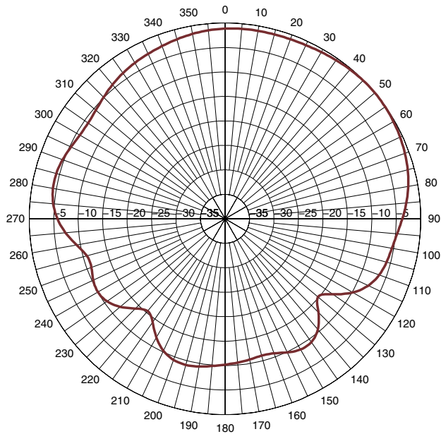
H-PLANE_960MHZ
