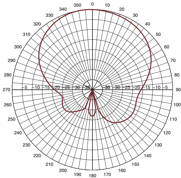
H-PLANE_2100MHZ
