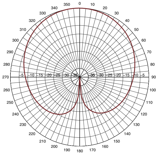
H-PLANE_698MHZ
