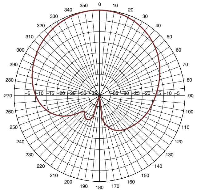
V-PLANE_698MHZ
