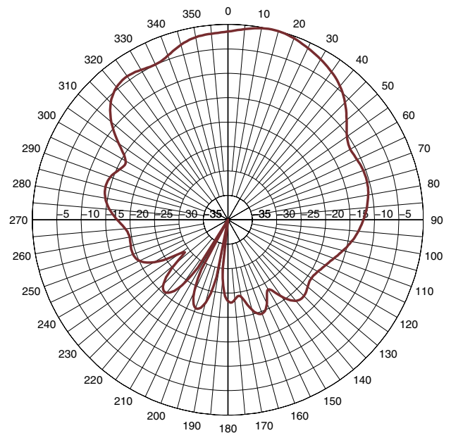
V-PLANE_2700MHZ
