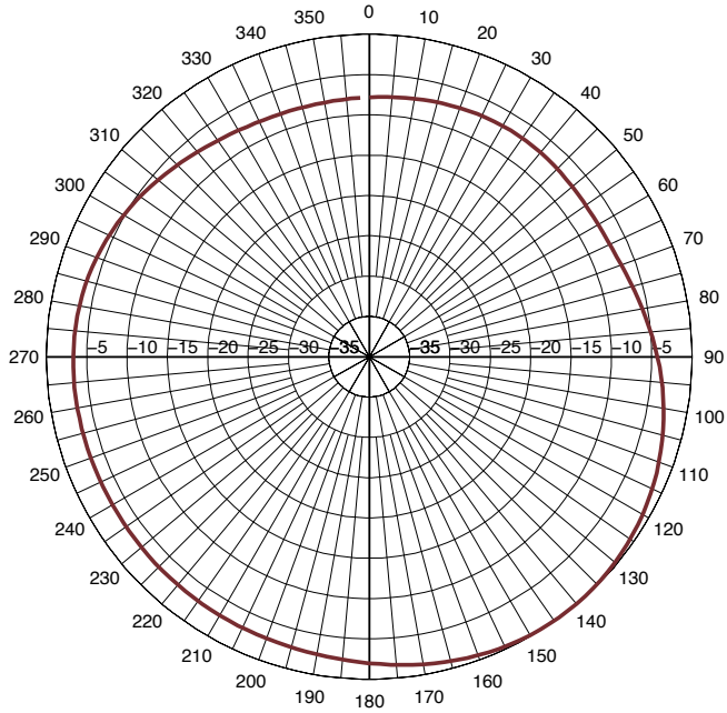
2 GHz-H-plane
