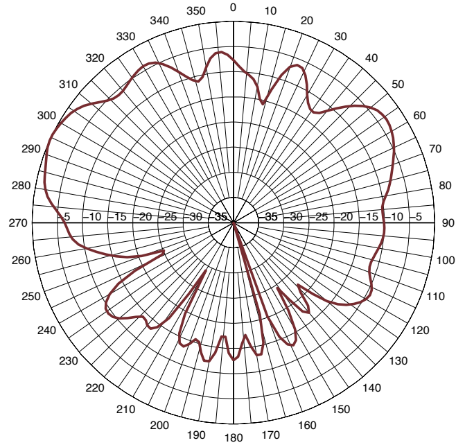
2 GHz-V-plane
