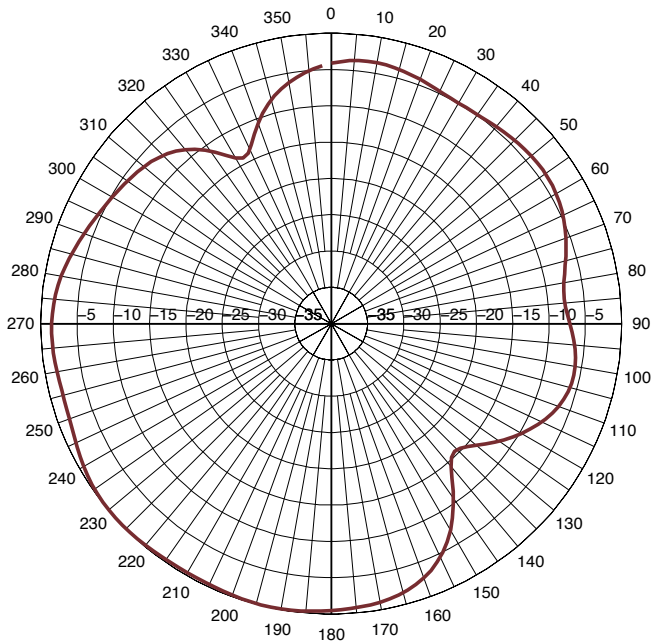
5 GHz-H-plane
