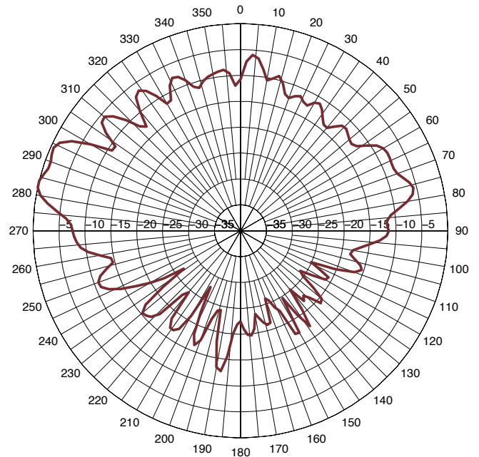
5 GHz-V-plane
